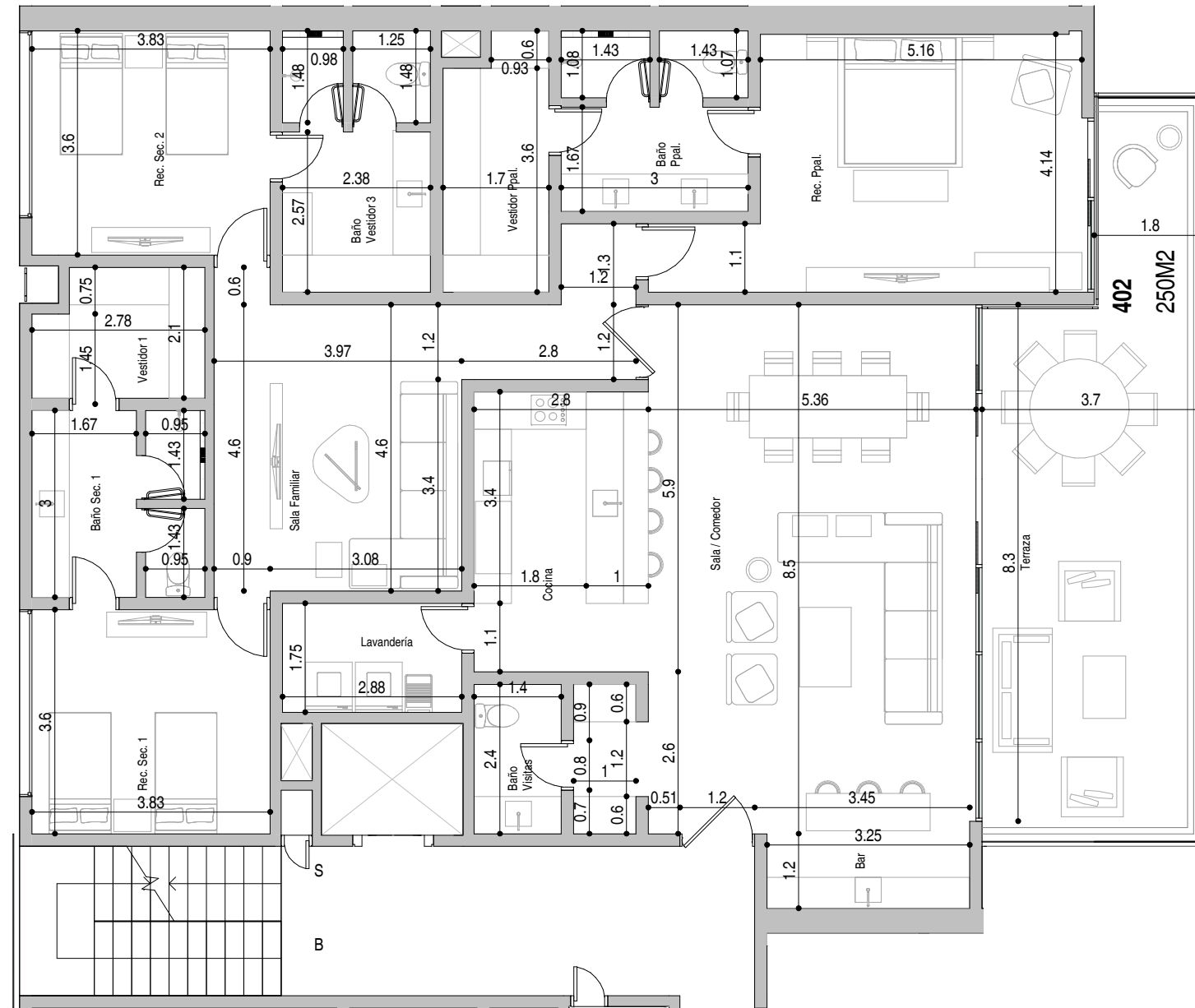
1 DEPARTAMENTO 402 1 : 100
