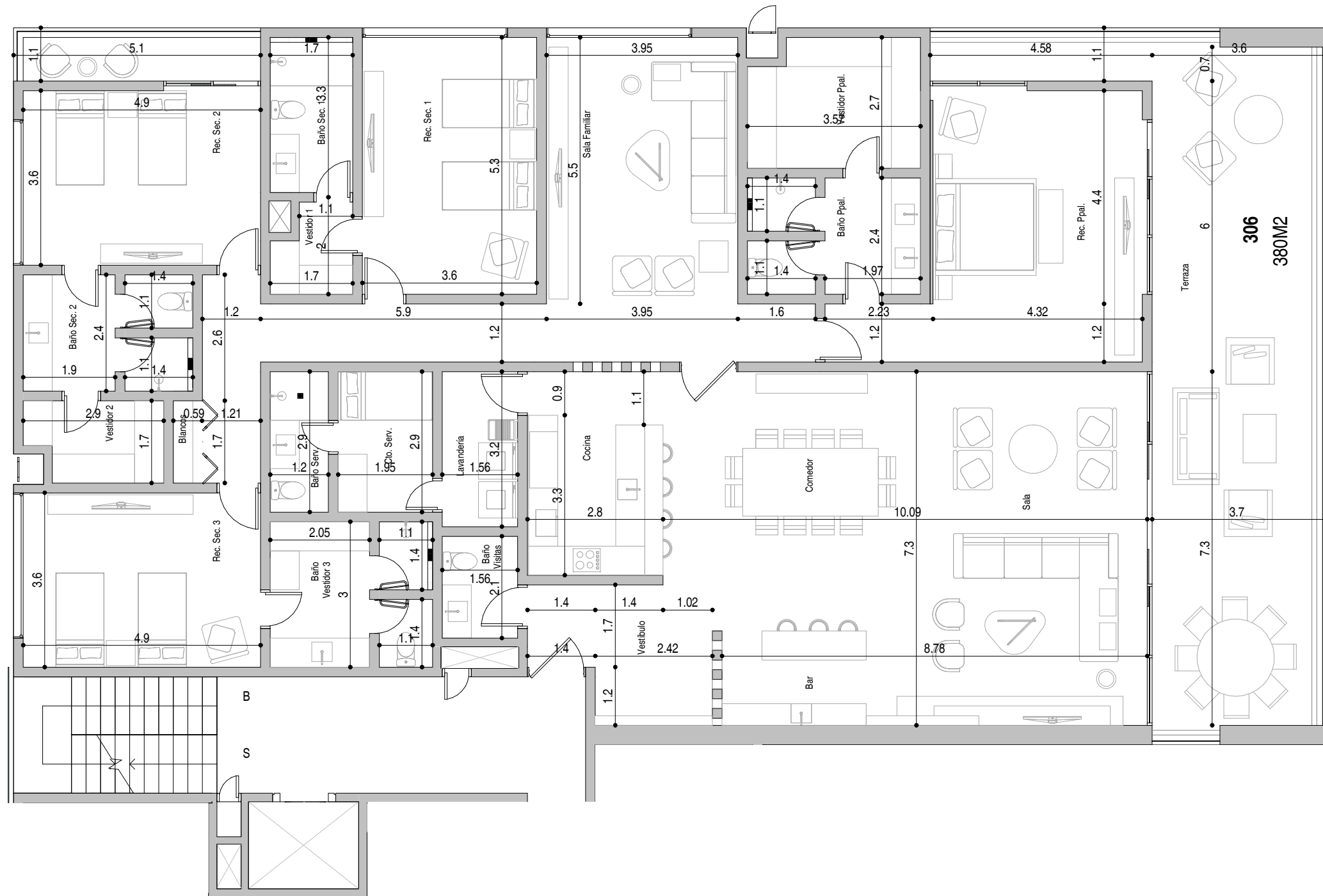
1 DEPARTAMENTO 306 1 : 100
