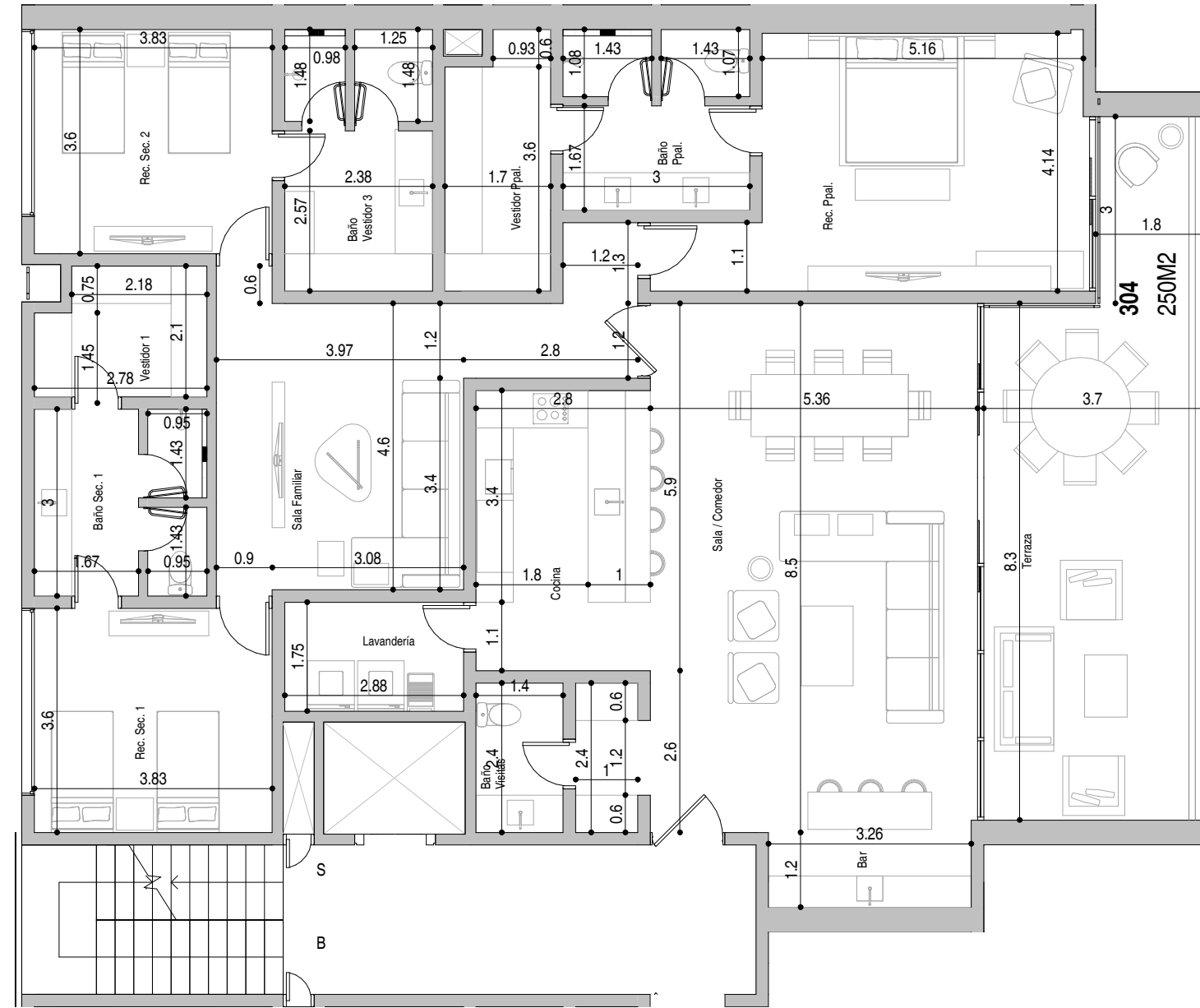
1 DEPARTAMENTO 304 1 : 100
