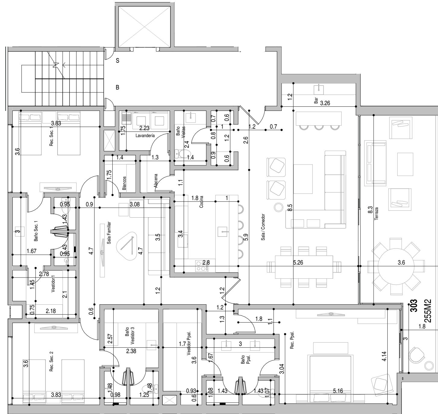
1 DEPARTAMENTO 303 1 : 100
