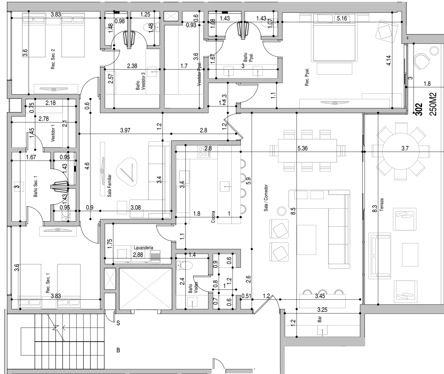
1 DEPARTAMENTO 302 1:100
