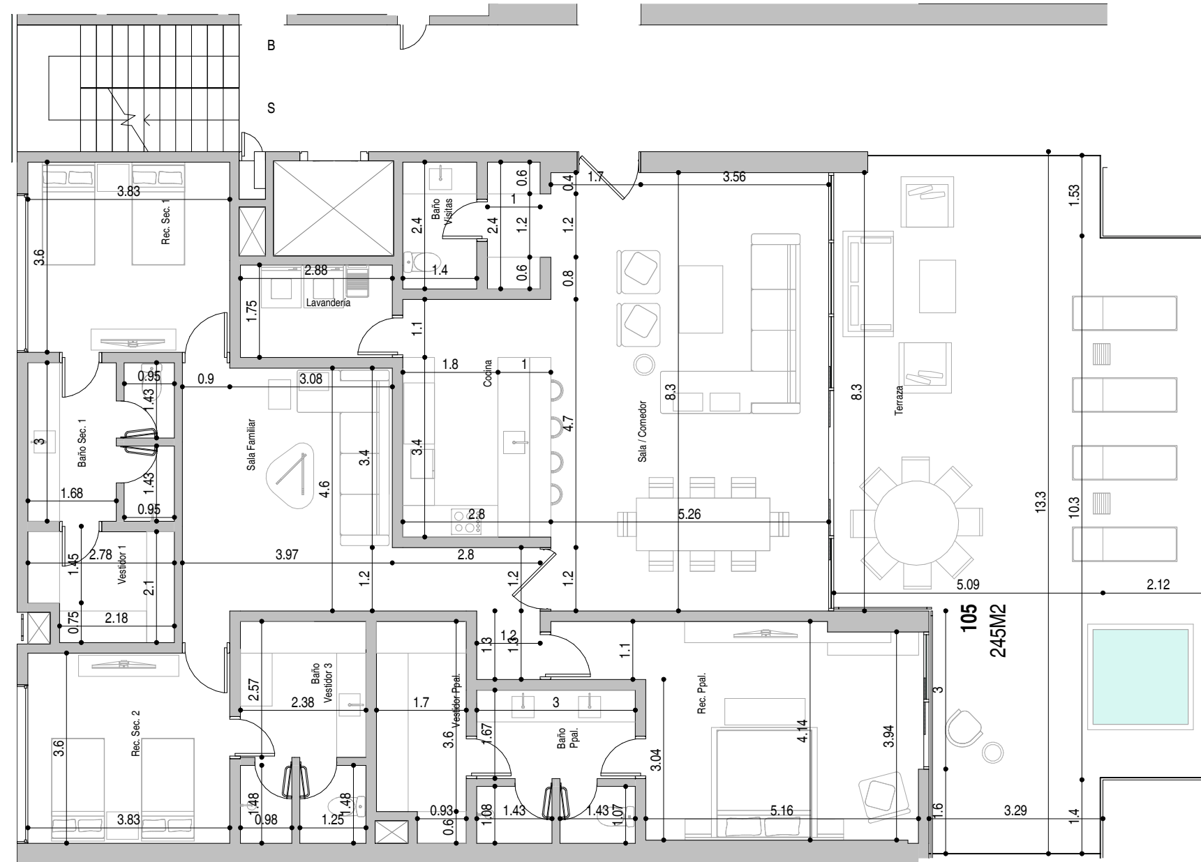
1 DEPARTAMENTO 105 1 : 100
